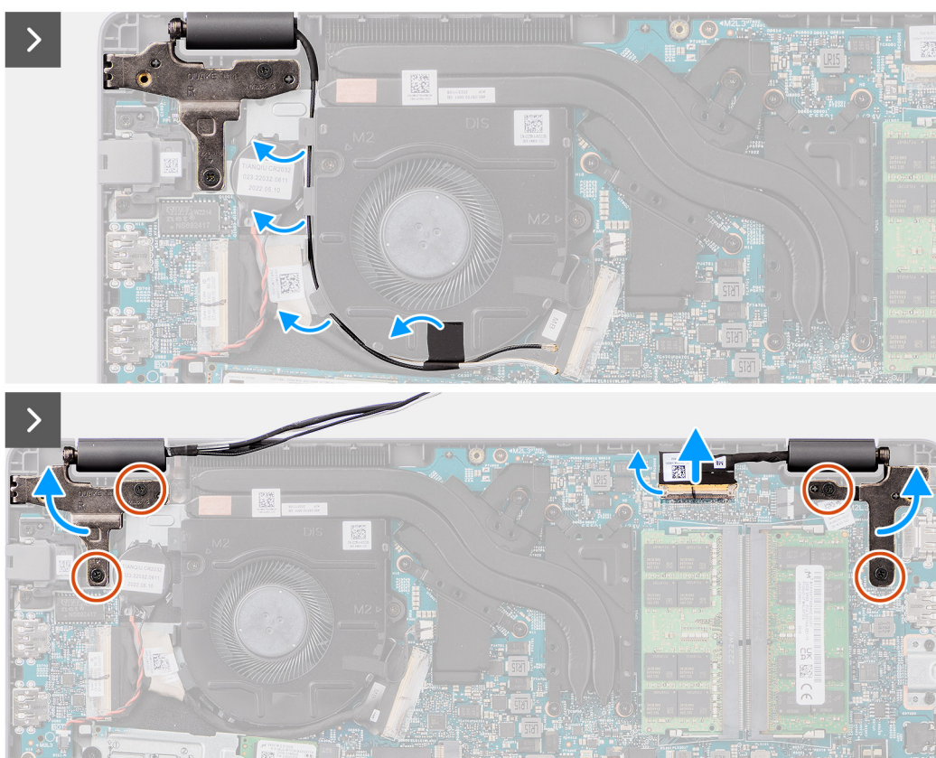
Rysunek 47. Wymontowywanie zestawu wyświetlacza
