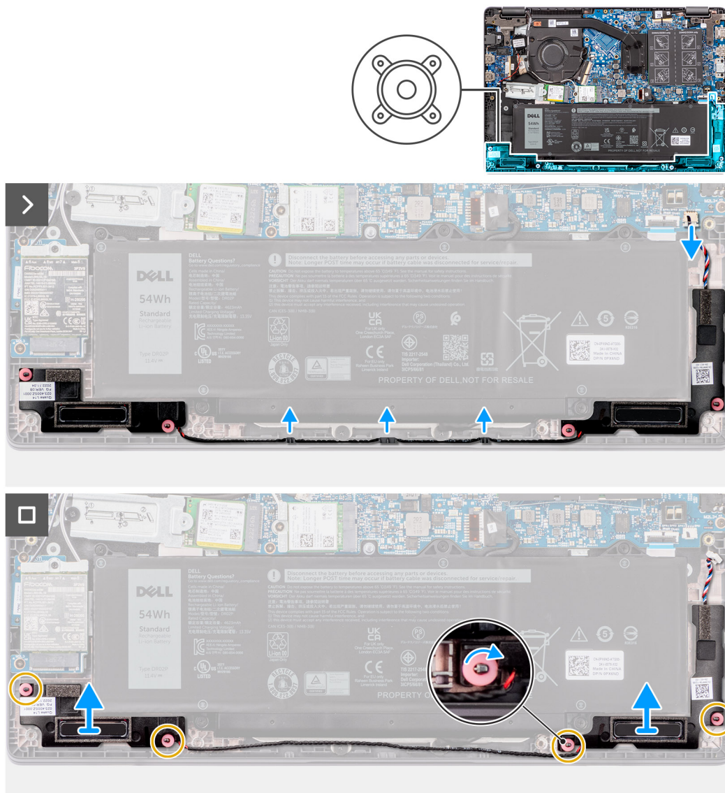
Rysunek 21. Wymontowywanie głośników
