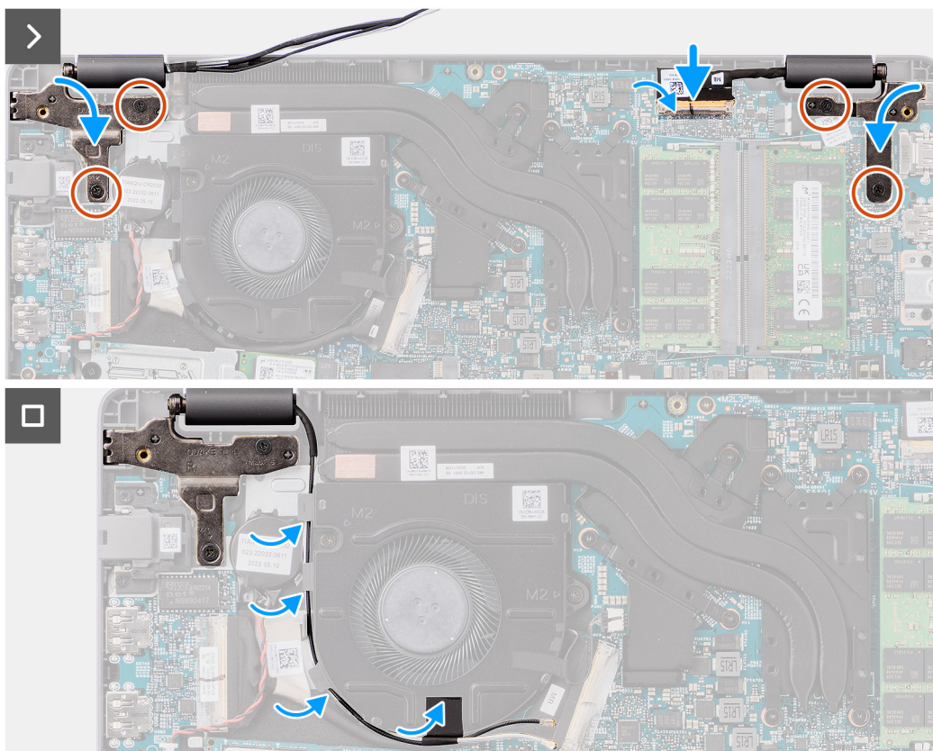
Rysunek 51. Instalowanie zestawu wyświetlacza
