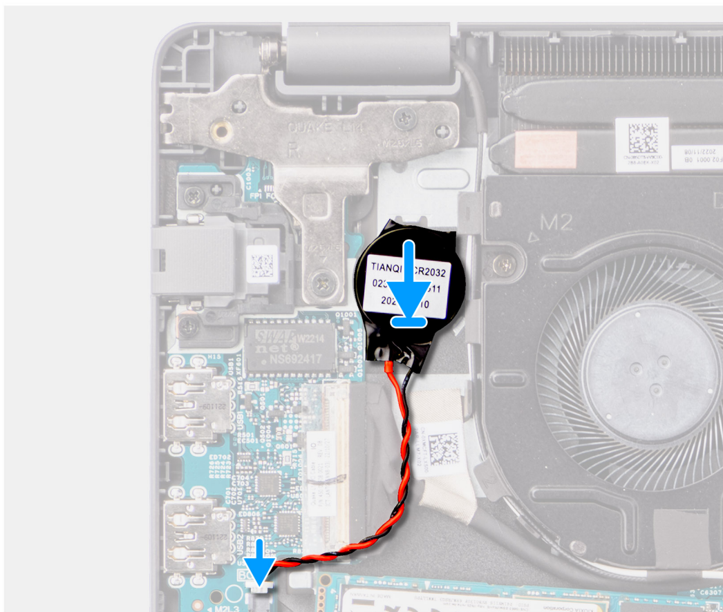
Rysunek 18. Instalowanie baterii pastylkowej
