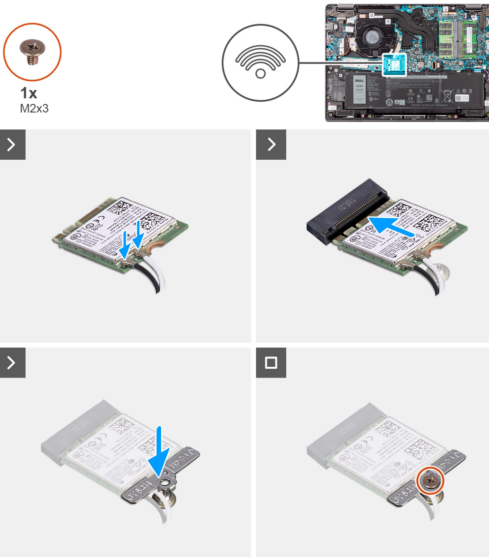
Rysunek 16. Instalowanie karty sieci bezprzewodowej
