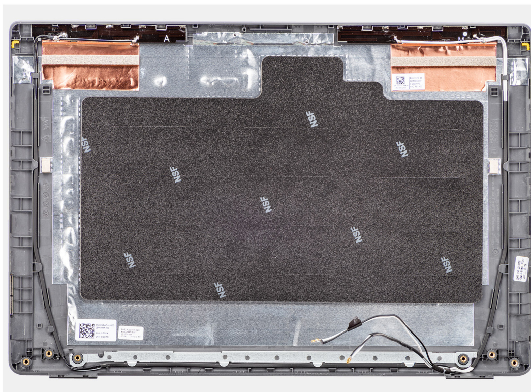
Rysunek 69. Instalowanie pokrywy tylnej wyświetlacza
