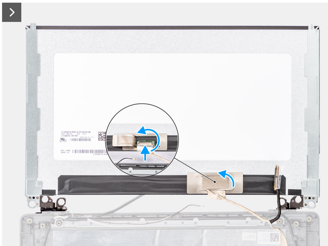
Rysunek 60. Instalowanie wyświetlacza
