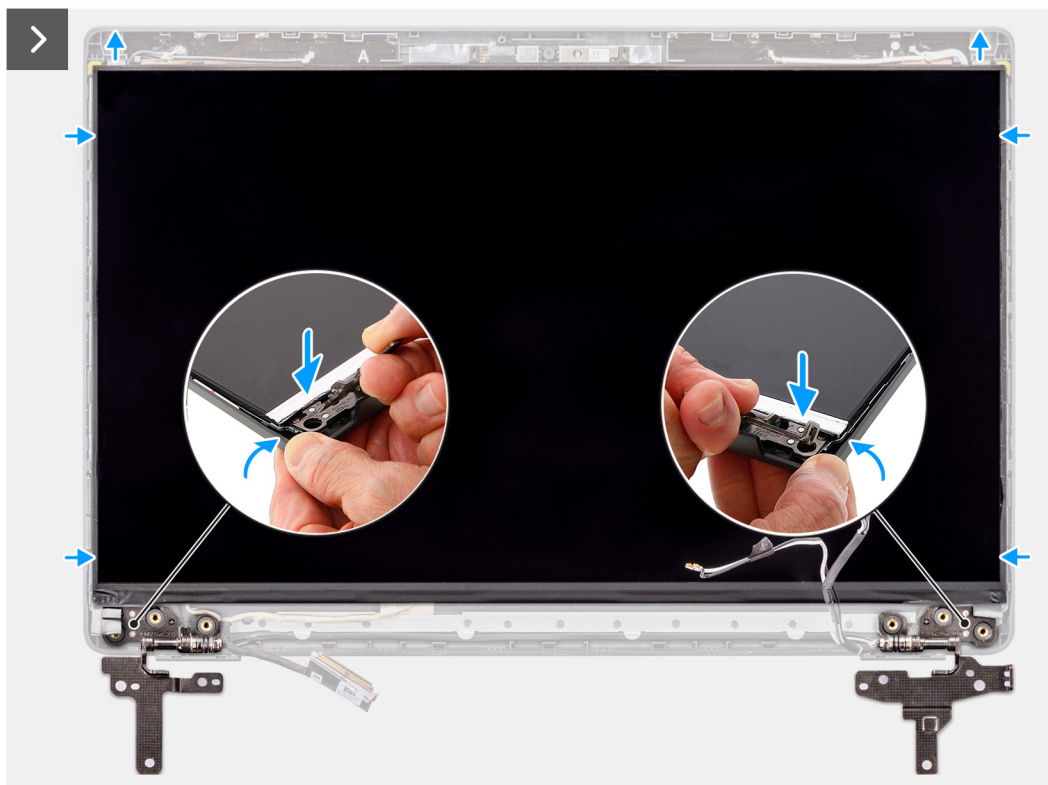
Rysunek 62. Instalowanie wyświetlacza
