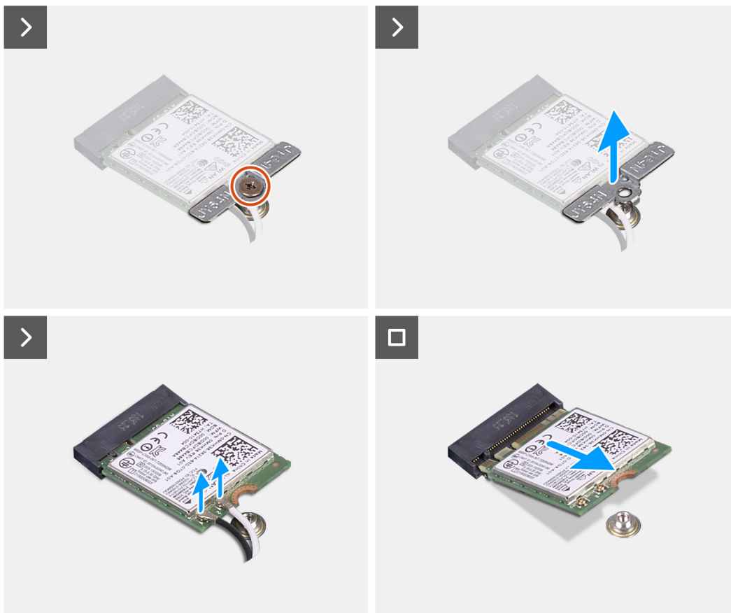
Rysunek 15. Wymontowywanie karty sieci bezprzewodowej
