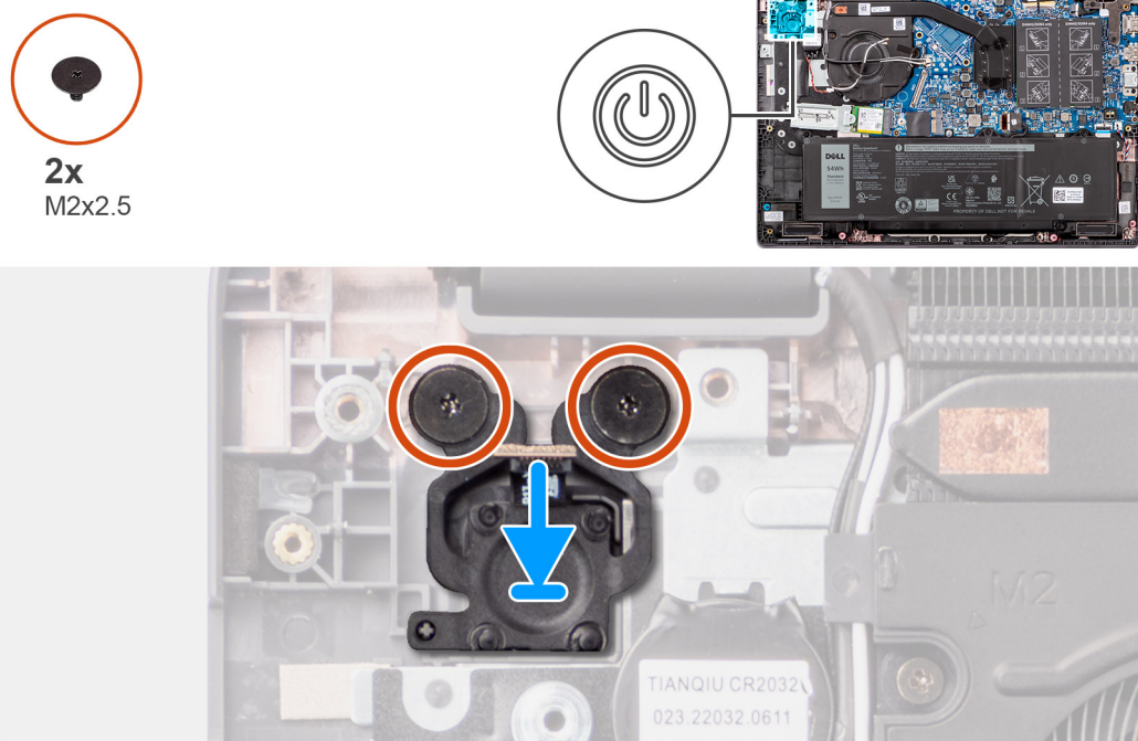
Rysunek 40. Instalowanie przycisku zasilania
