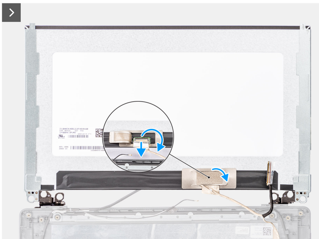
Rysunek 57. Wymontowywanie wyświetlacza
