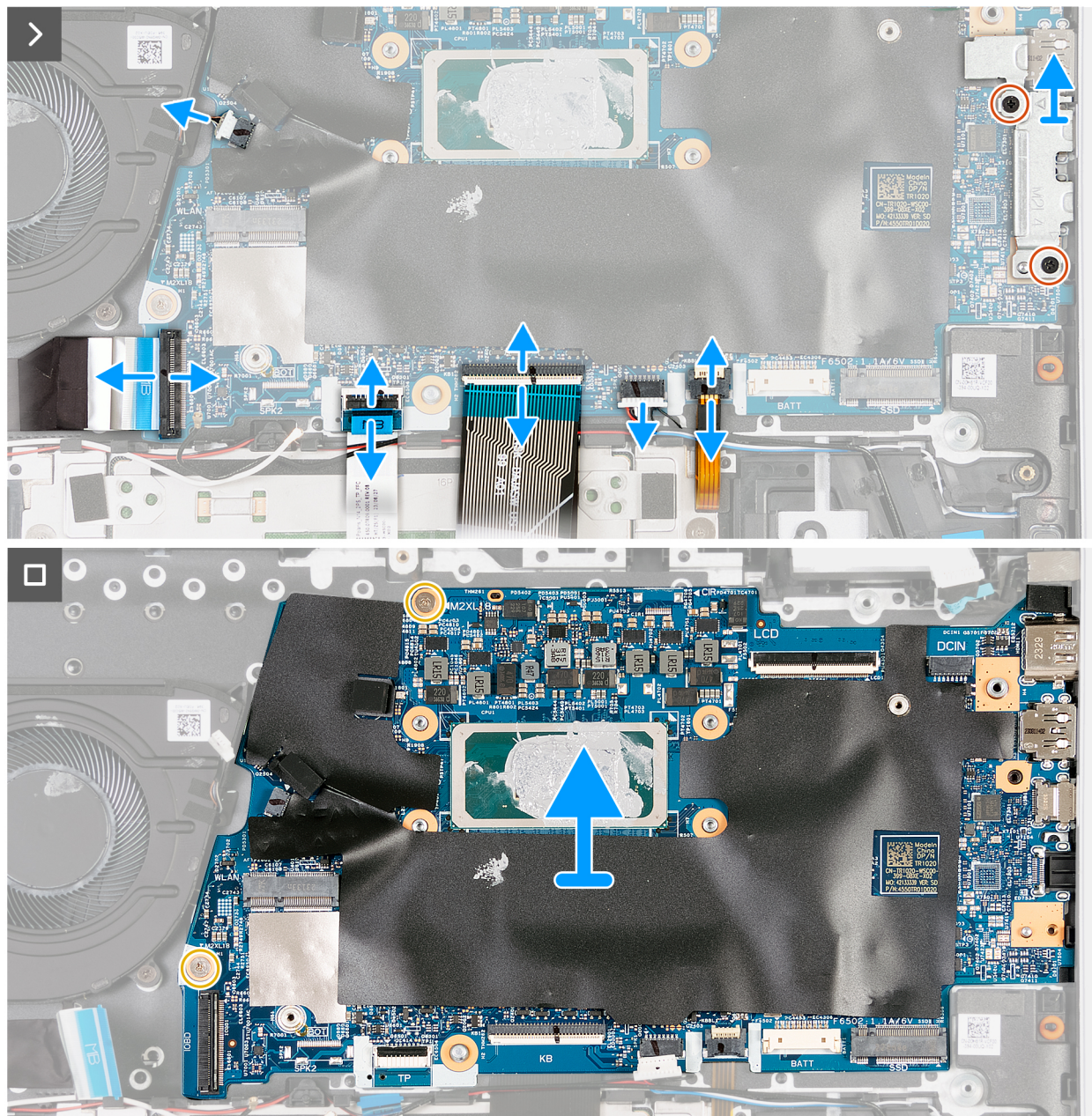
Rysunek 37. Wymontowywanie płyty głównej
