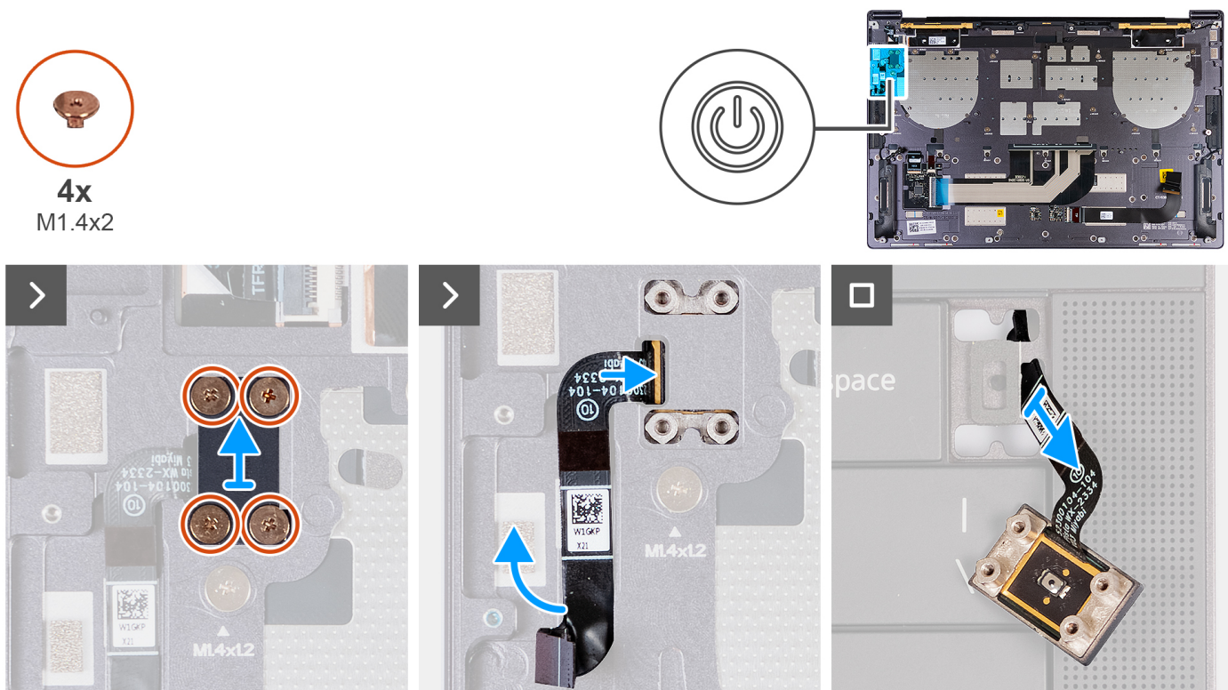
Rysunek 37. Wymontowywanie przycisku zasilania z czytnikiem linii papilarnych
