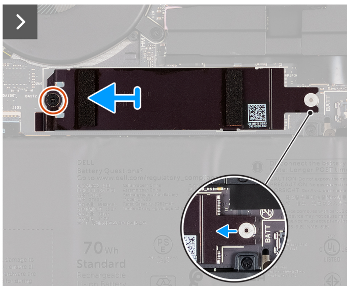
Rysunek 21. Wymontowywanie dysku SSD M.2 2280
