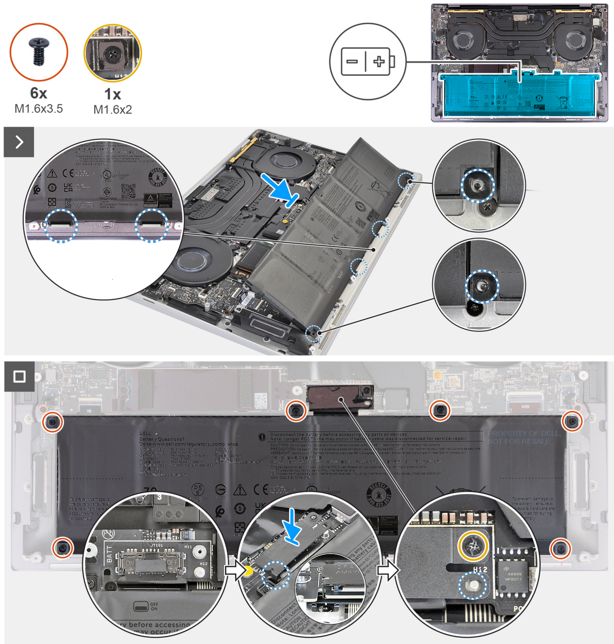
Rysunek 17. Instalowanie baterii
