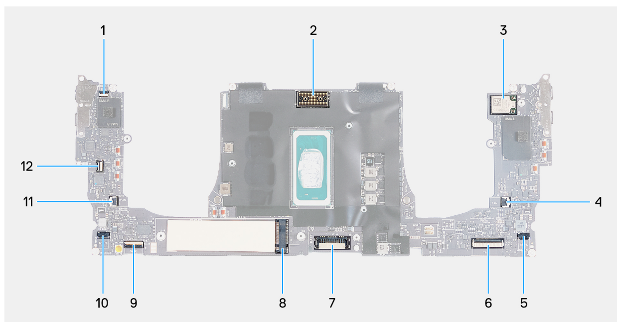
Rysunek 34. Złącza płyty głównej
