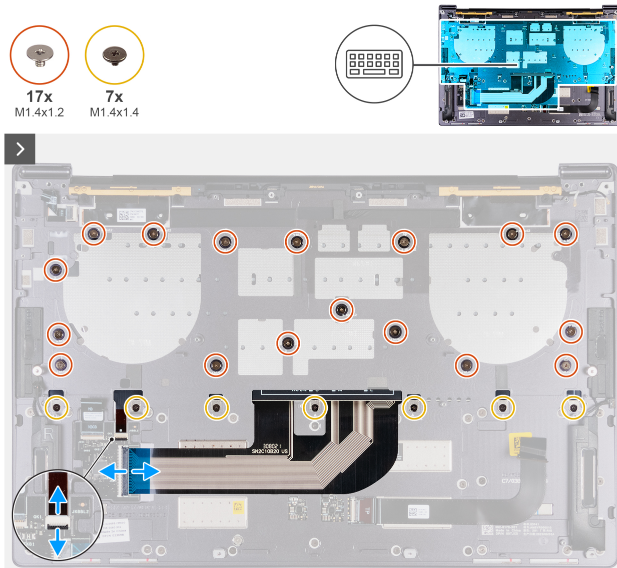
Rysunek 40. Wymontowywanie klawiatury
