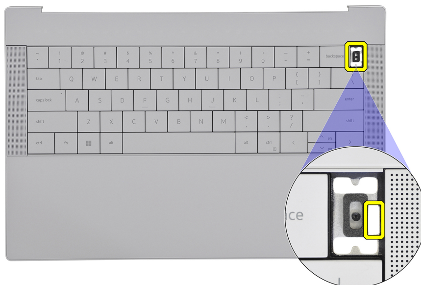
Rysunek 38. Przycisk zasilania z czytnikiem linii papilarnych
