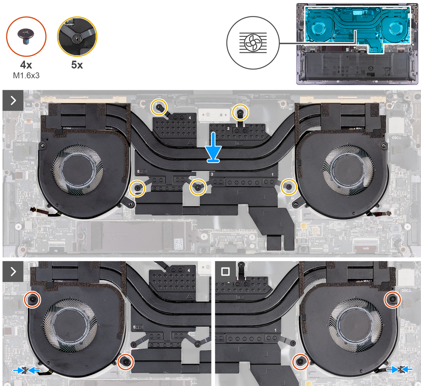
Rysunek 25. Instalowanie zestawu radiatora
