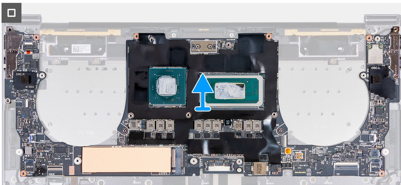
Rysunek 33. Wymontowywanie płyty głównej
