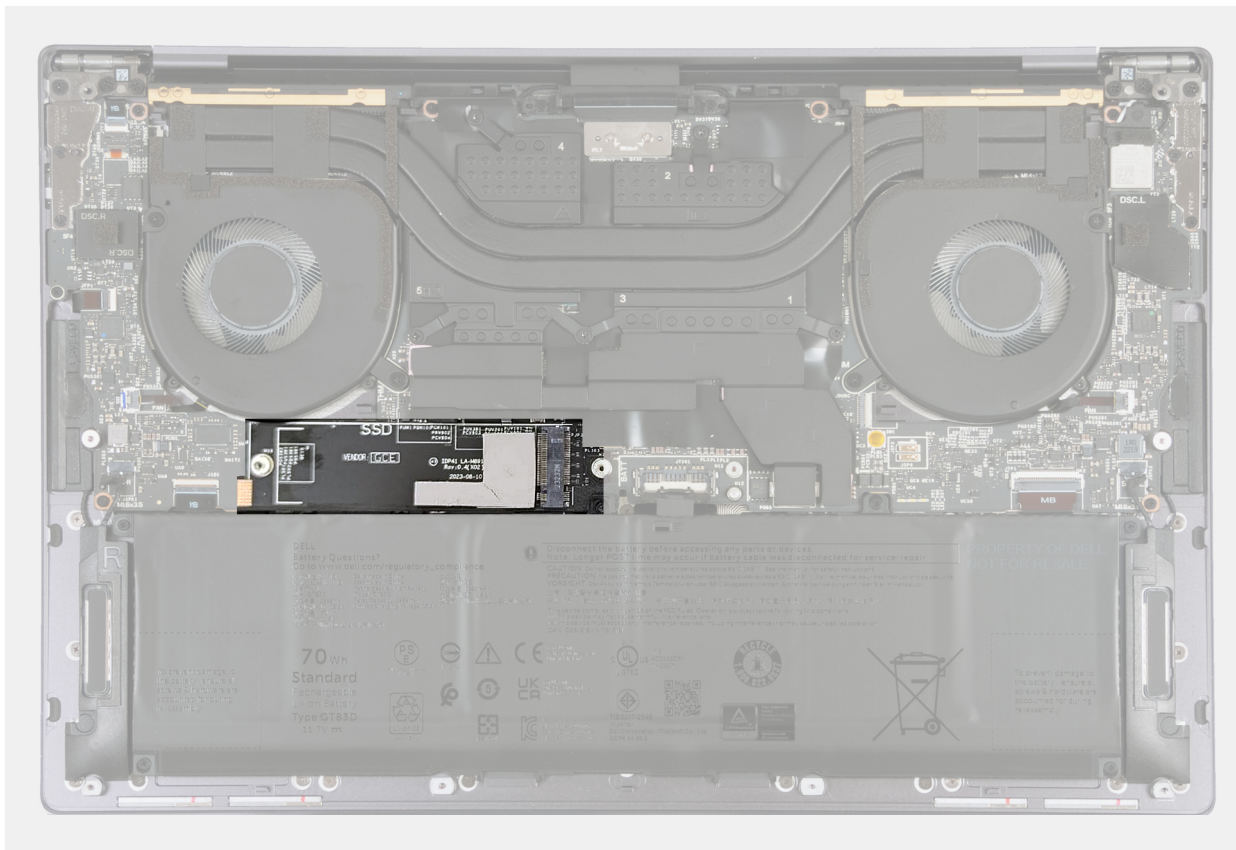
Rysunek 22. Podkładka termoprzewodząca dysku SSD M.2
