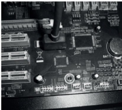
Umieszczenie w porcie 3.0 na płycie głównej
